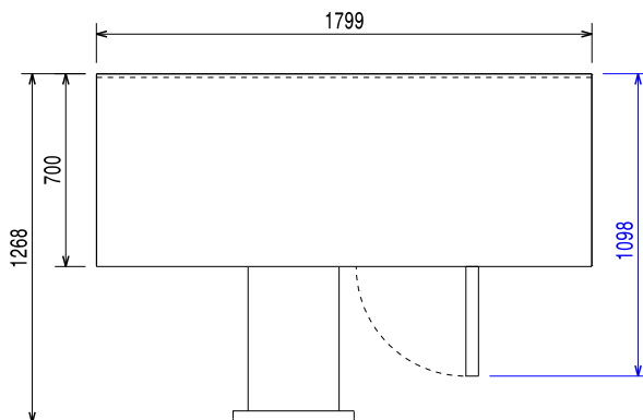
Boven aanzicht
